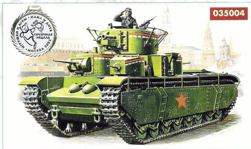
Советский тяжёлый танк Т-35
