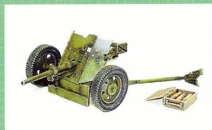
45-мм Советская противотанковая пушка образца 1938/42 года
